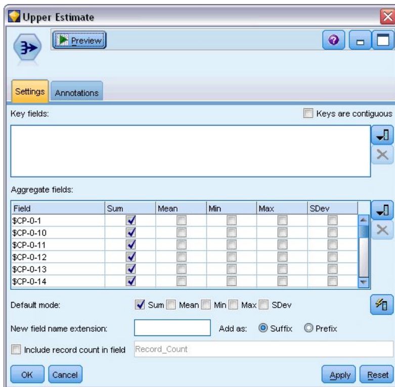
Figura 362. Nodo Agregar: pestaña Configuración
