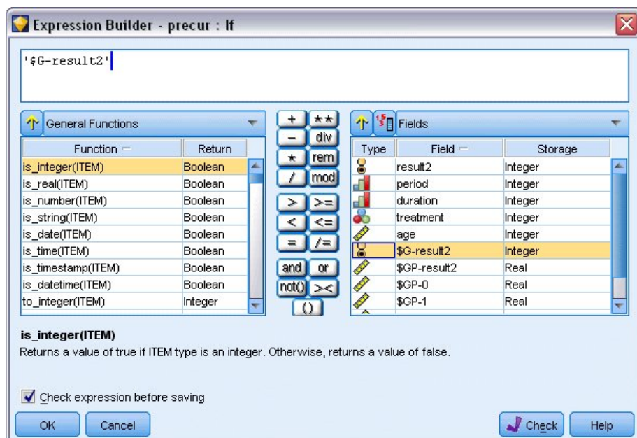
Figura 305. Nodo Derivar: Generador de expresiones de la condición Si
