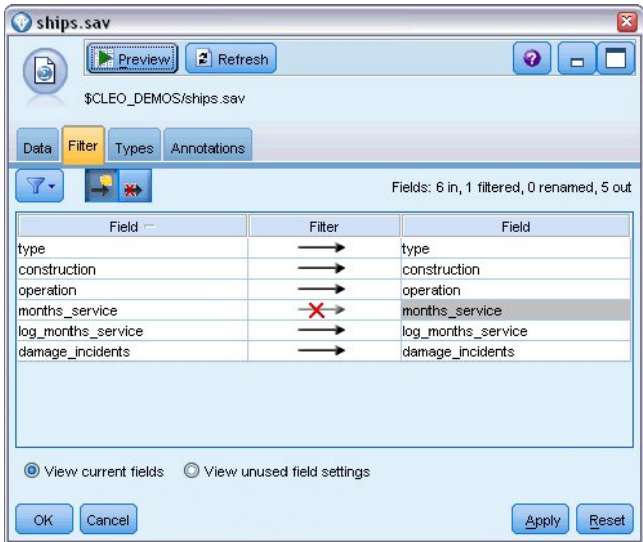
Figura 311. Filtrado de un campo innecesario
