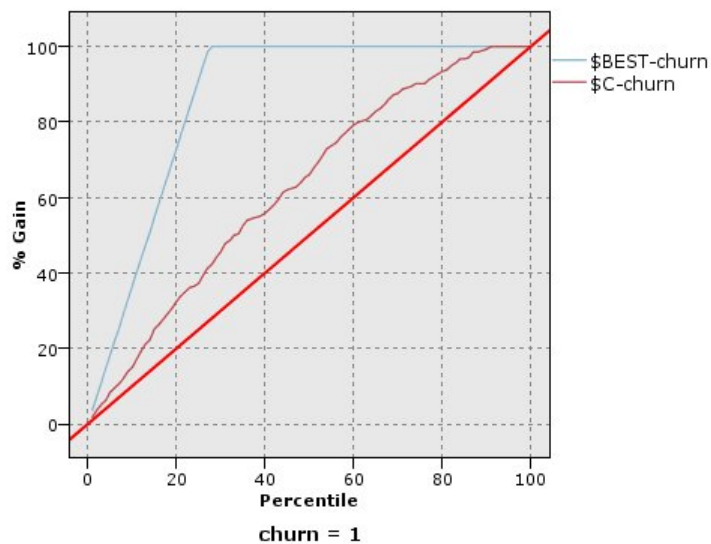
Figura 356. Gráfico de ganancias
