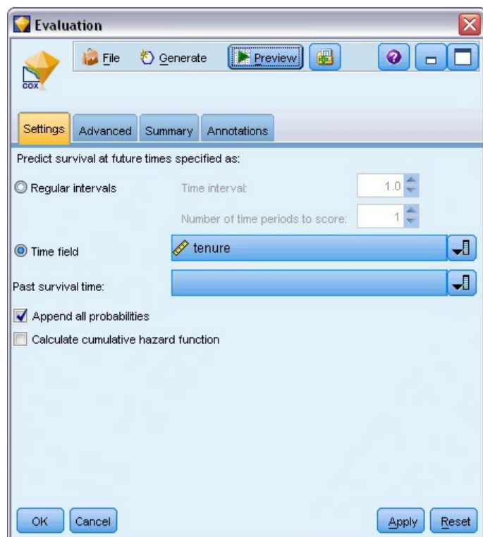
Figura 353. Nugget de Cox: pestaña Configuración
