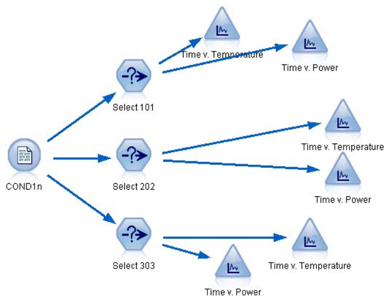
Figura 260. Ruta condplot
