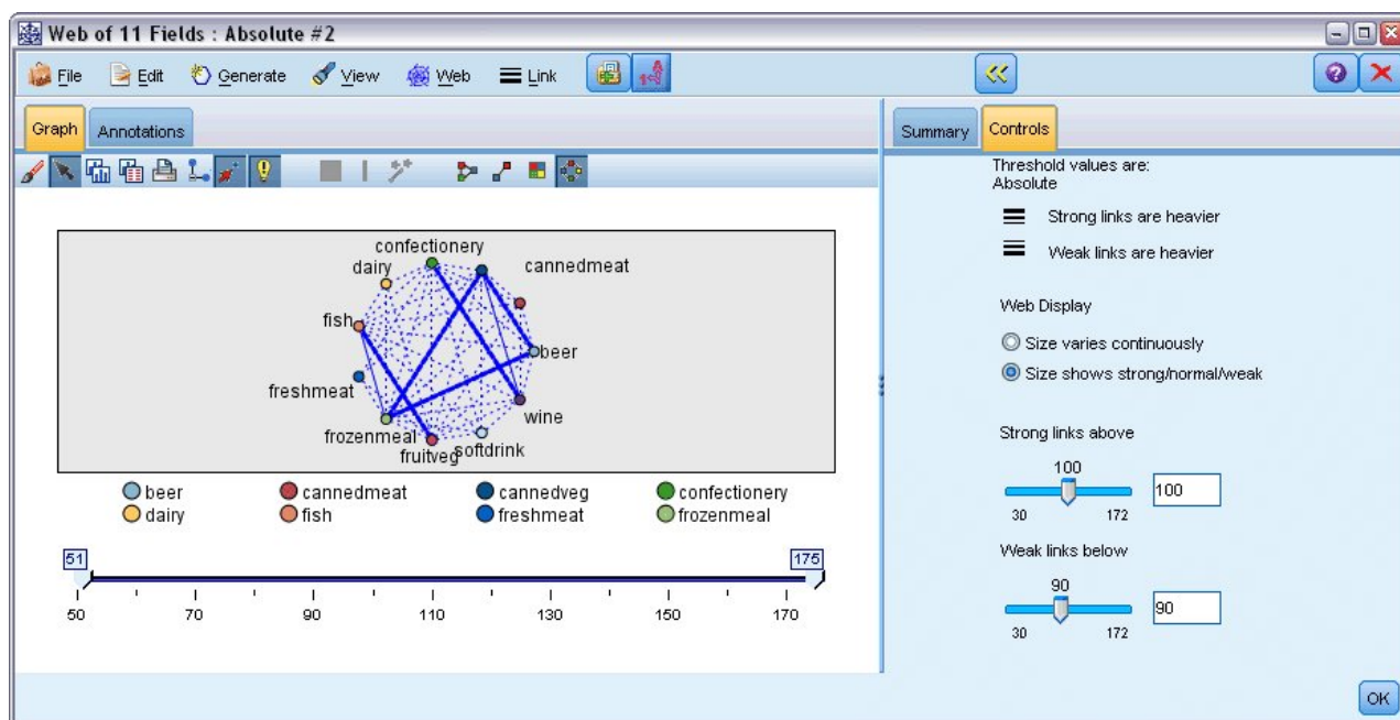
Figura 384. Visualización de malla restringida
