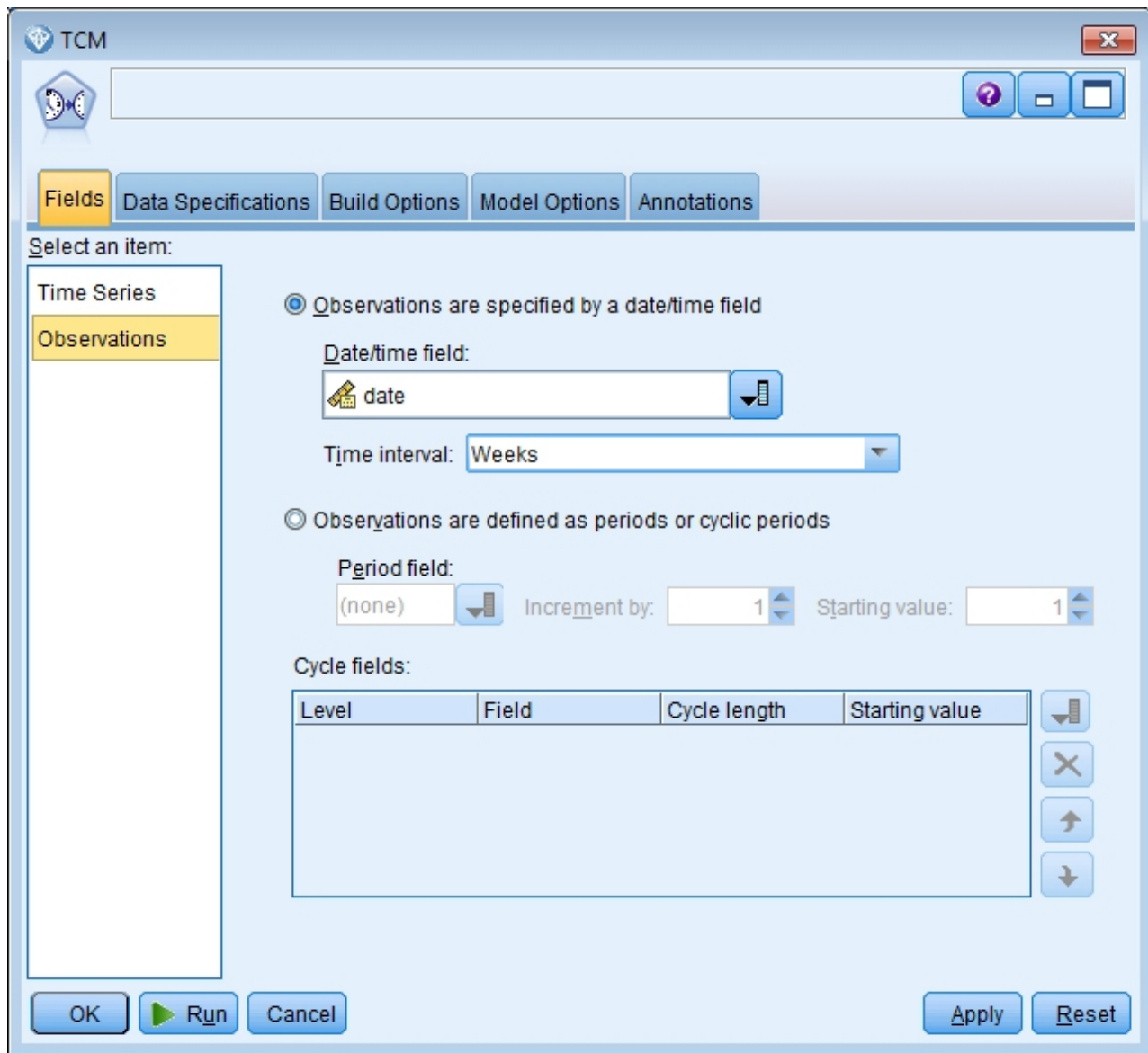
Figura 399. Modelado causal temporal, observaciones
