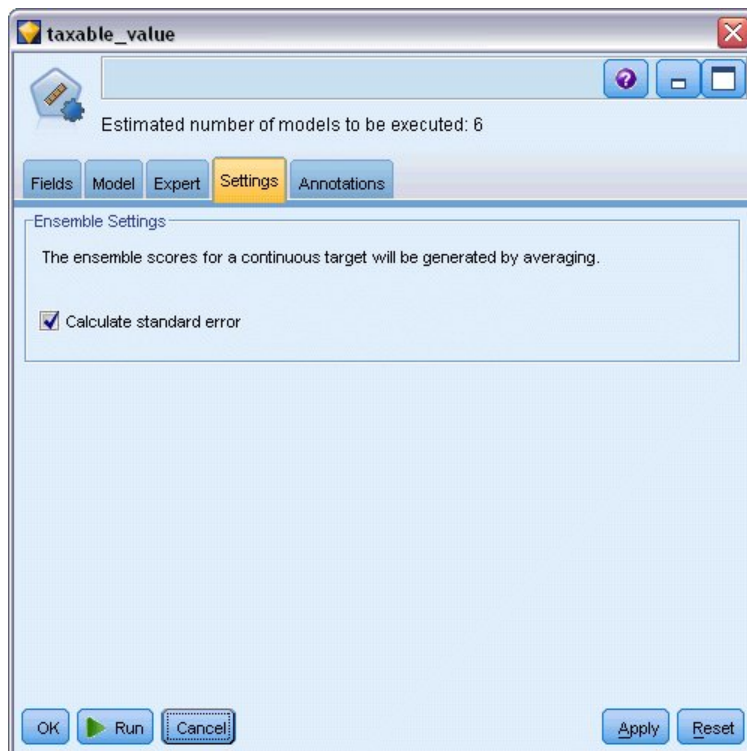
Figura 47. Pestaña Configuración del nodo Autonumérico
