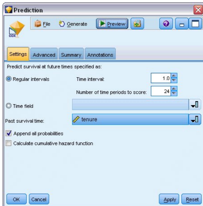
Figura 359. Nugget de Cox: pestaña Configuración
