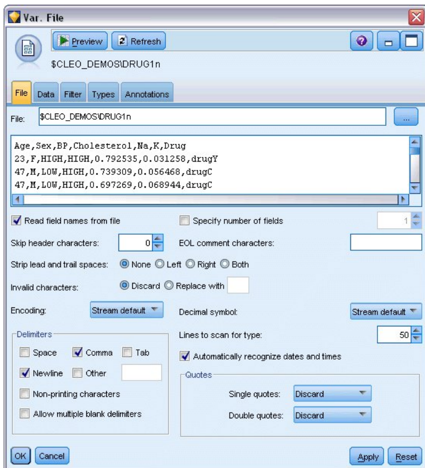
Figura 78. Cuadro de diálogo Archivo var.
