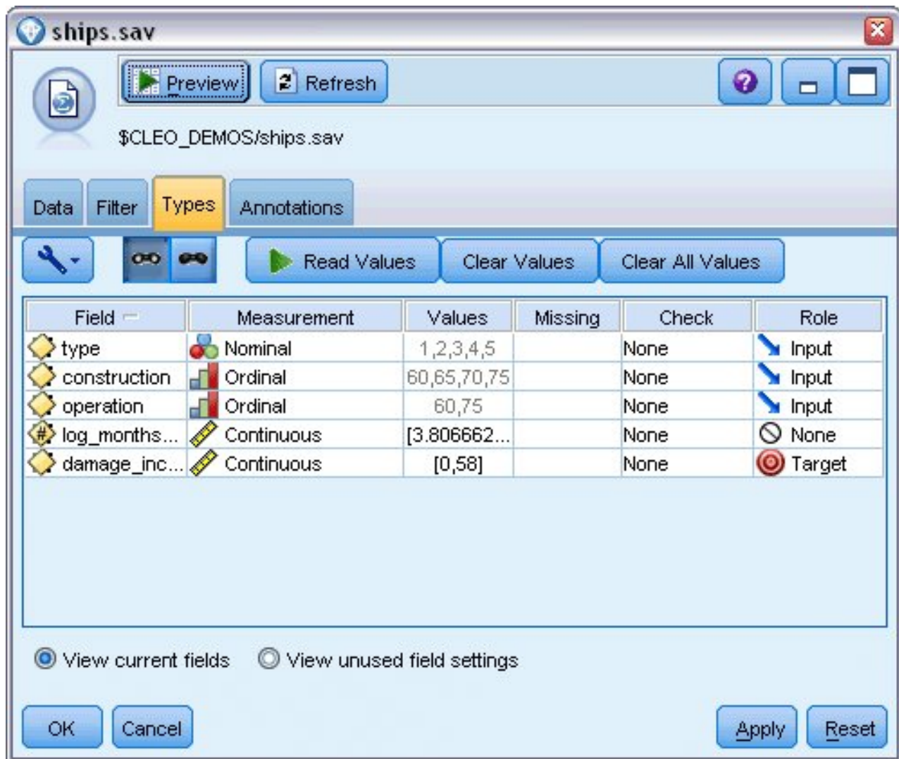
Figura 312. Definición del rol de campos
