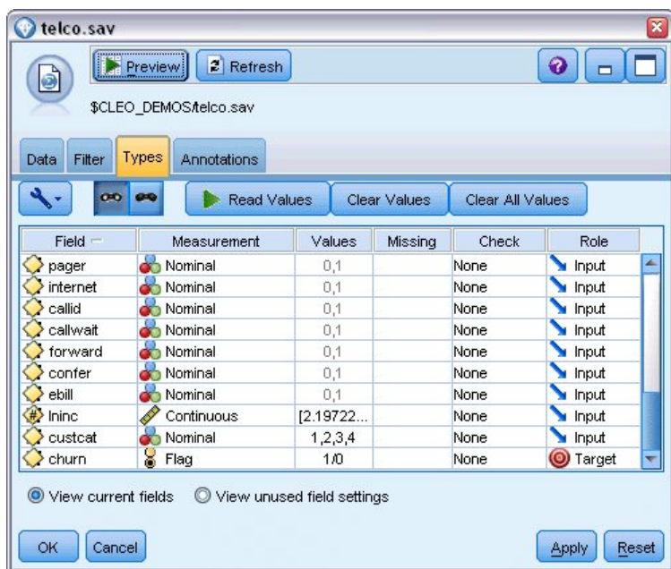
Figura 341. Definición del rol de campos
