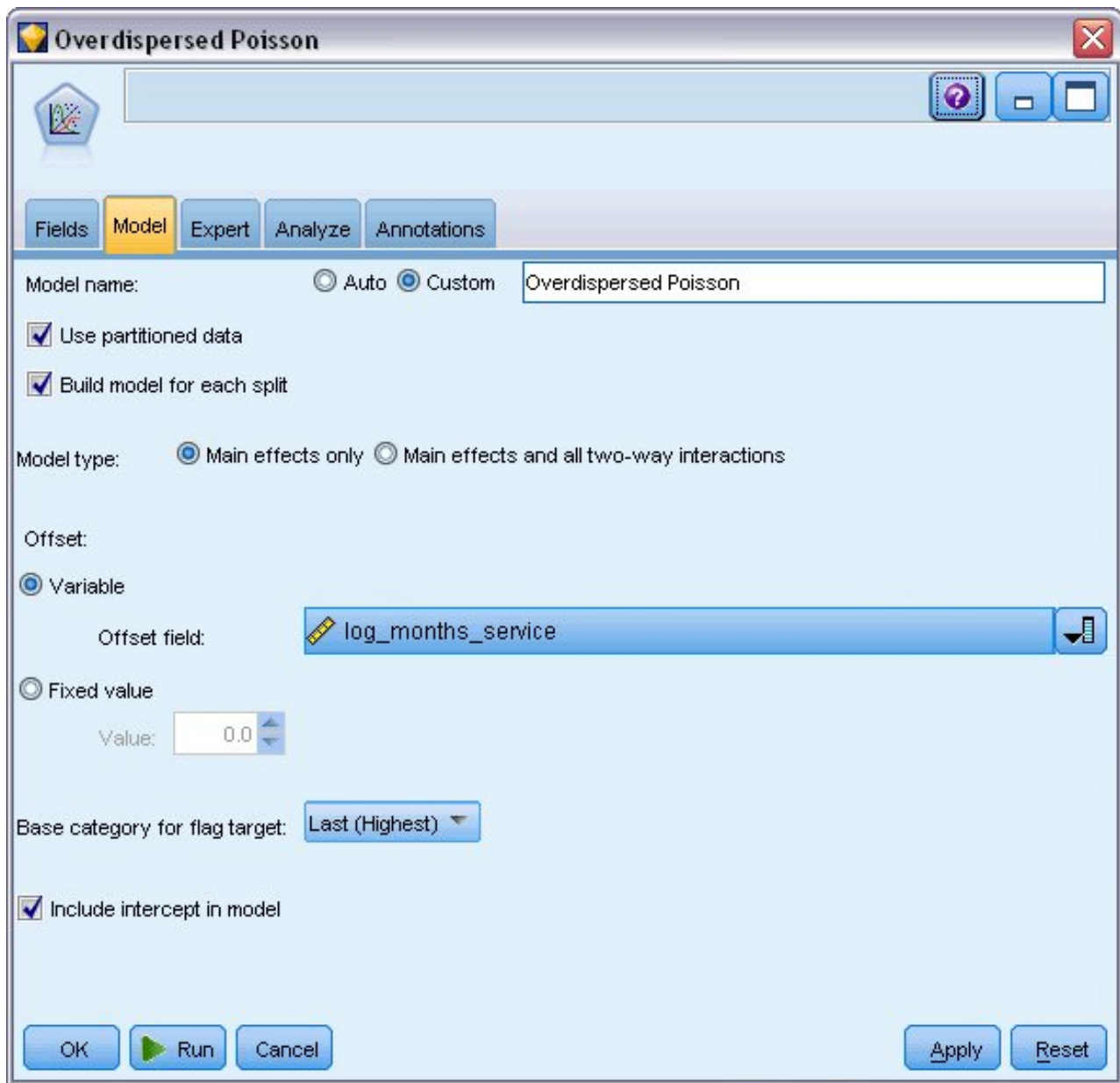
Figura 313. Selección de opciones del modelo
