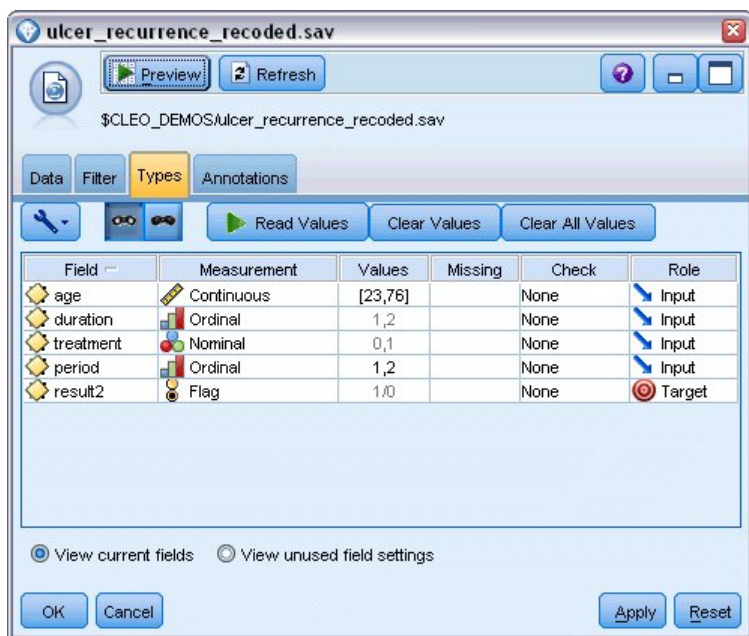
Figura 297. Definición del rol de campos
