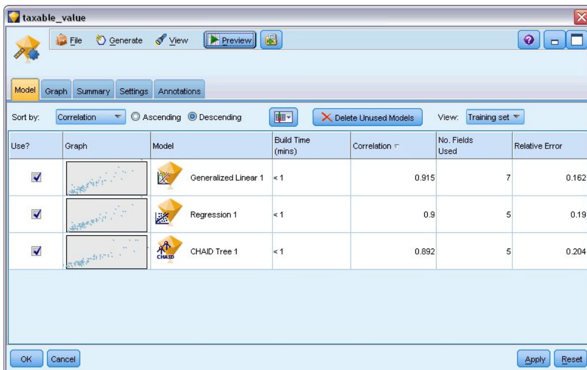
Figura 48. Resultados Autonuméricos
